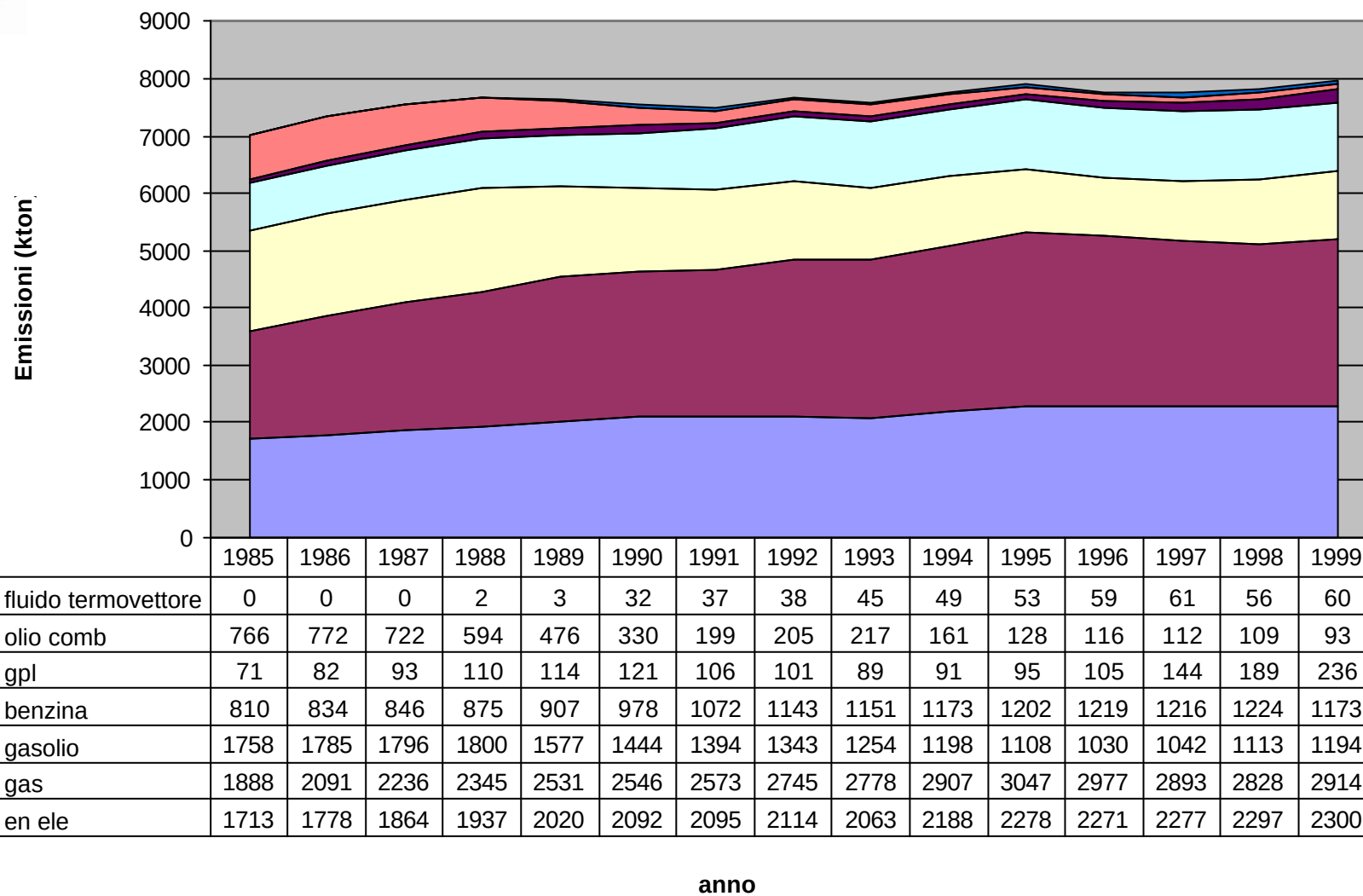
Grafico D.2.3.4: Emissioni di CO2 equivalente per vettore energetico
