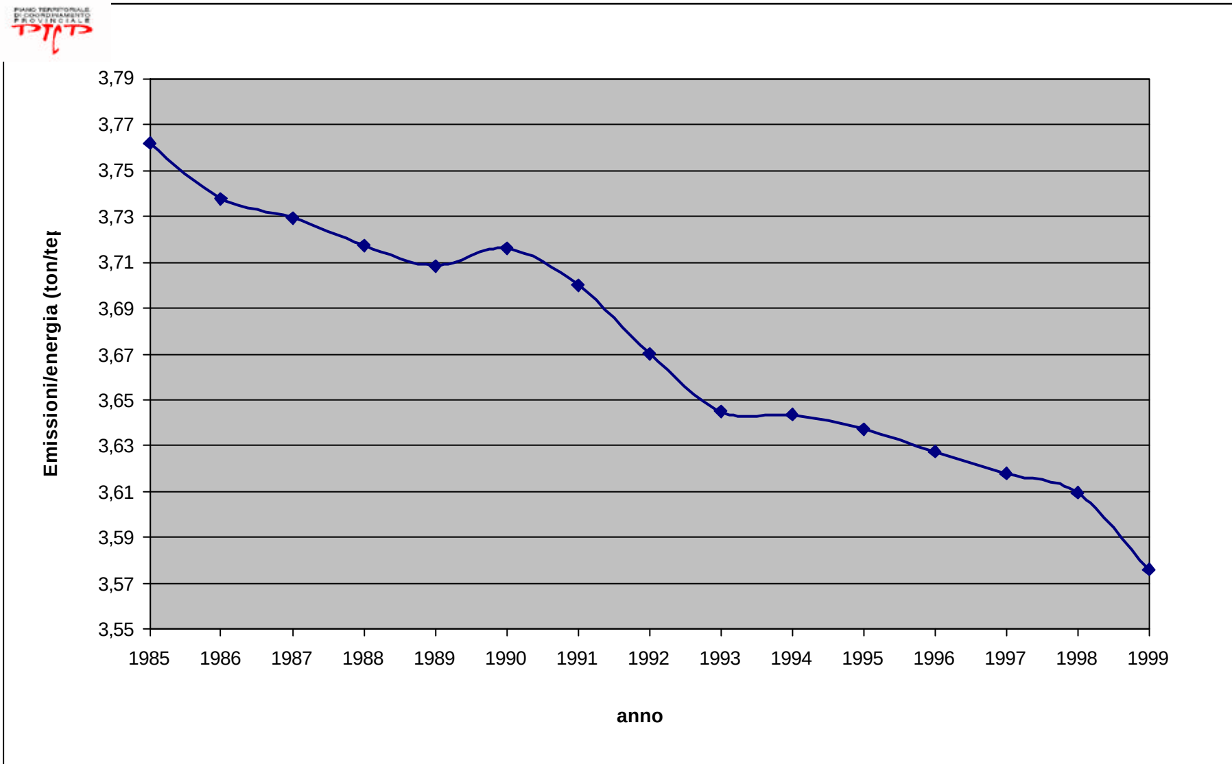
Grafico D.2.3.2: Andamento delle emissioni di CO2 equivalente per unità di energia consumata
